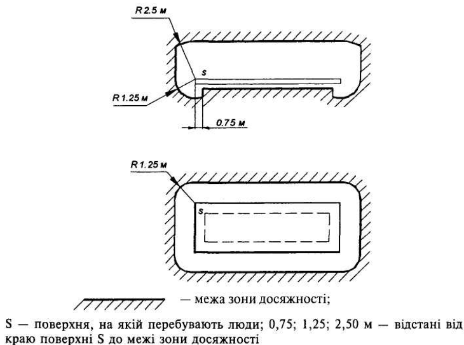
Рисунок 1.7.3 — Зони досяжності в електроустановках до 1 кВ
